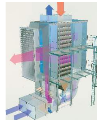
Heat exchanger KU Cooler 热交换器 KU 冷却器 Heat exchanger KS Cooler 热交换器 KS 冷却器
