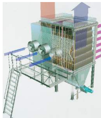
Heat exchanger KU Cooler 热交换器 KU 冷却器 Heat exchanger KS Cooler 热交换器 KS 冷却器
